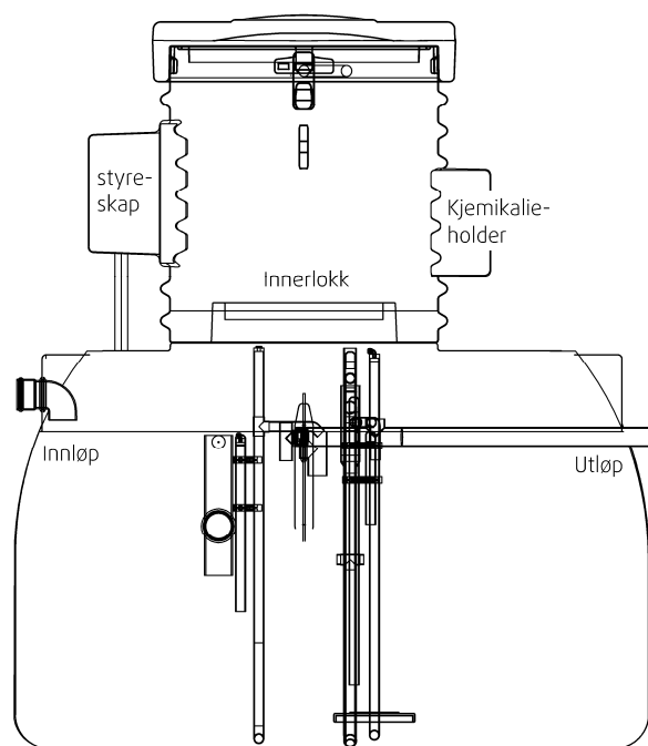
SNITT
